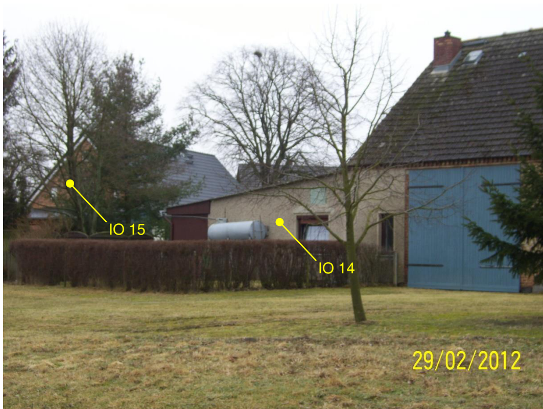
Bild 11: Wohngebäude Starow 20a (Südostfassade), Starow 21 (Ostfassade)
